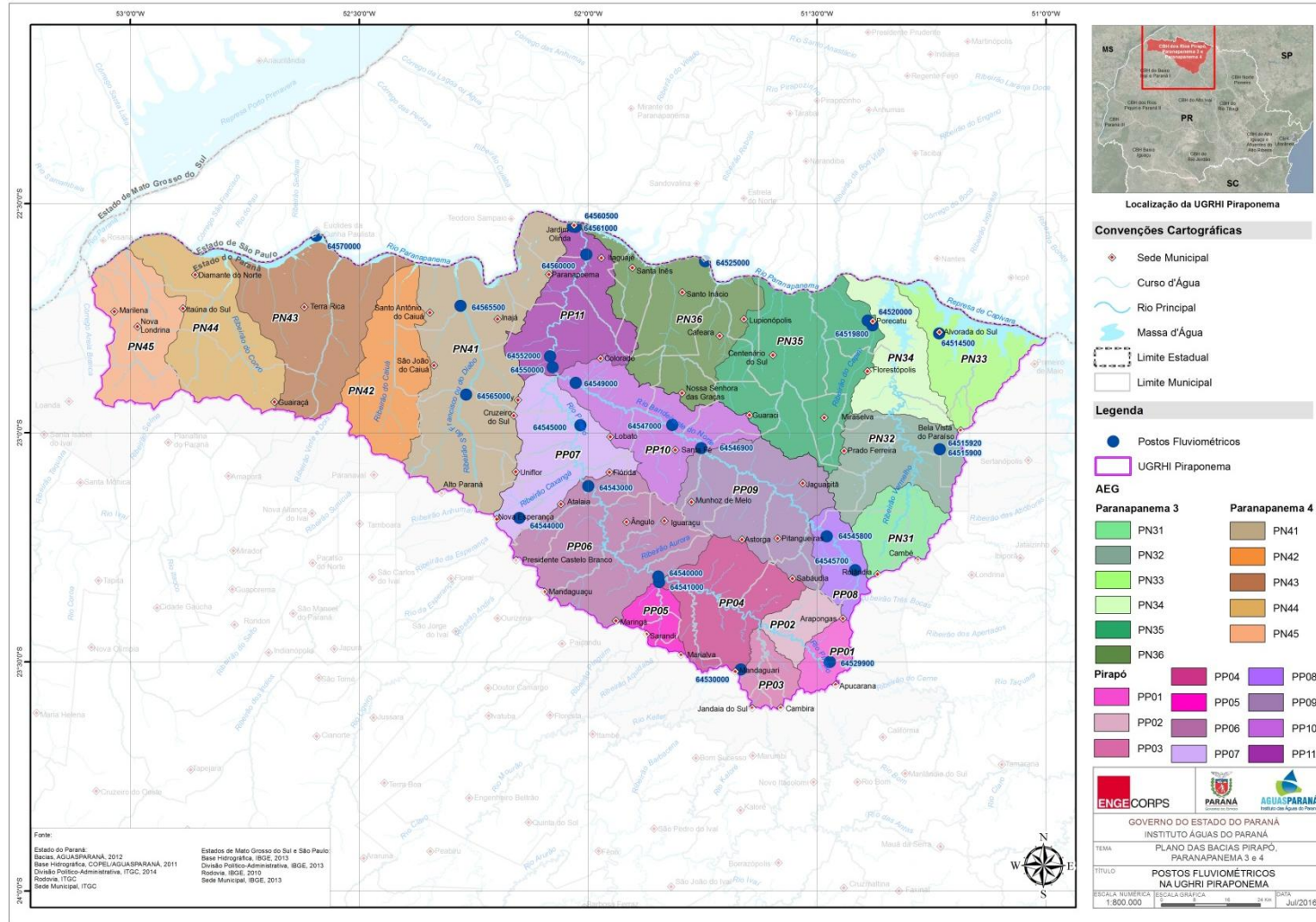
Figura 1.5 – Postos Fluviométricos na UGRHI Piraponema
