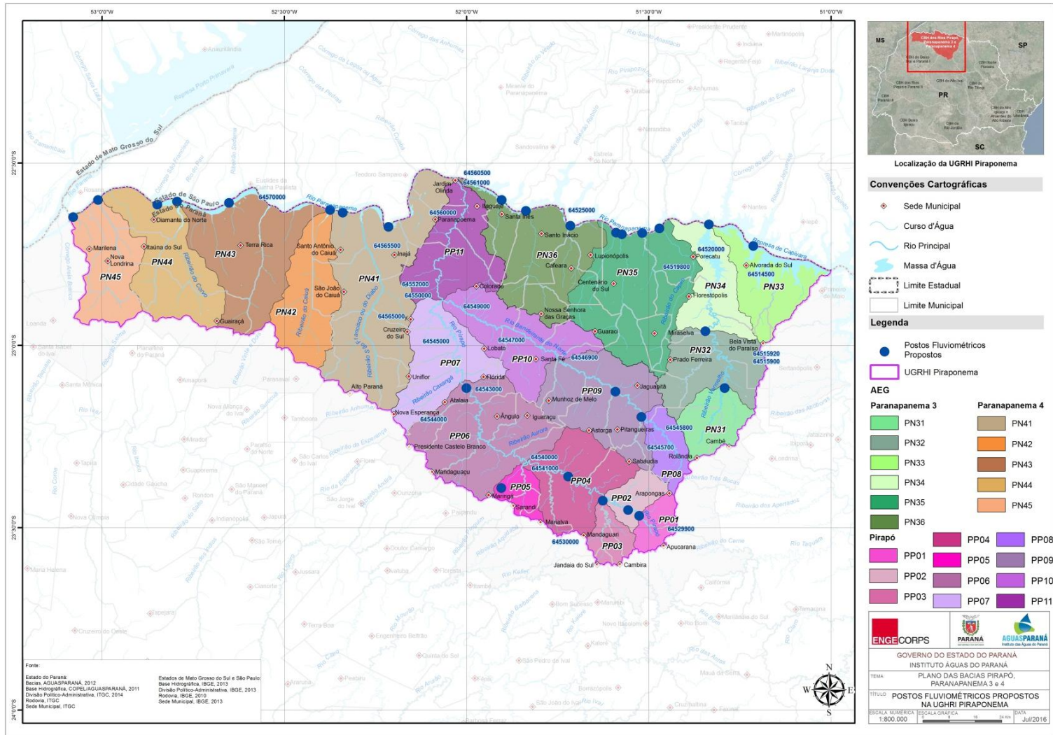
Figura 1.7 – Proposta de Rede de Monitoramento Fluviométrico da UGRHI Pirapomena
